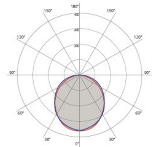
Courbe photométrique
